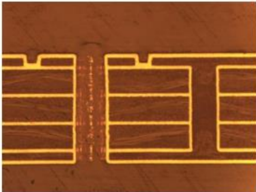
1阶HDI
